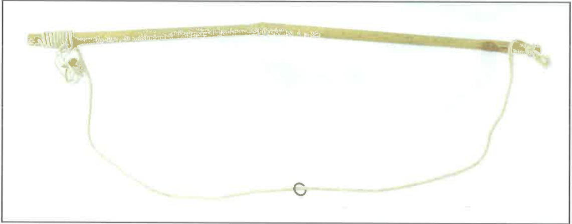
قوس لتدوير المجدح لثقب ألواح الخشب في جدار السفينة تمهيداً لوضع المسمار فيه .
